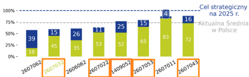
Penetracja lokalowa 100 Mb/s aktualna i po realizacji POPC na tle sąsiednich gmin
